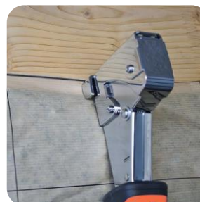
AGRAFADOR MARTELO GRAMPO - TIPO G
