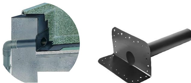
TUBO DE DESCARGA FRONTAL REDONDO EM PP+TPE-V
